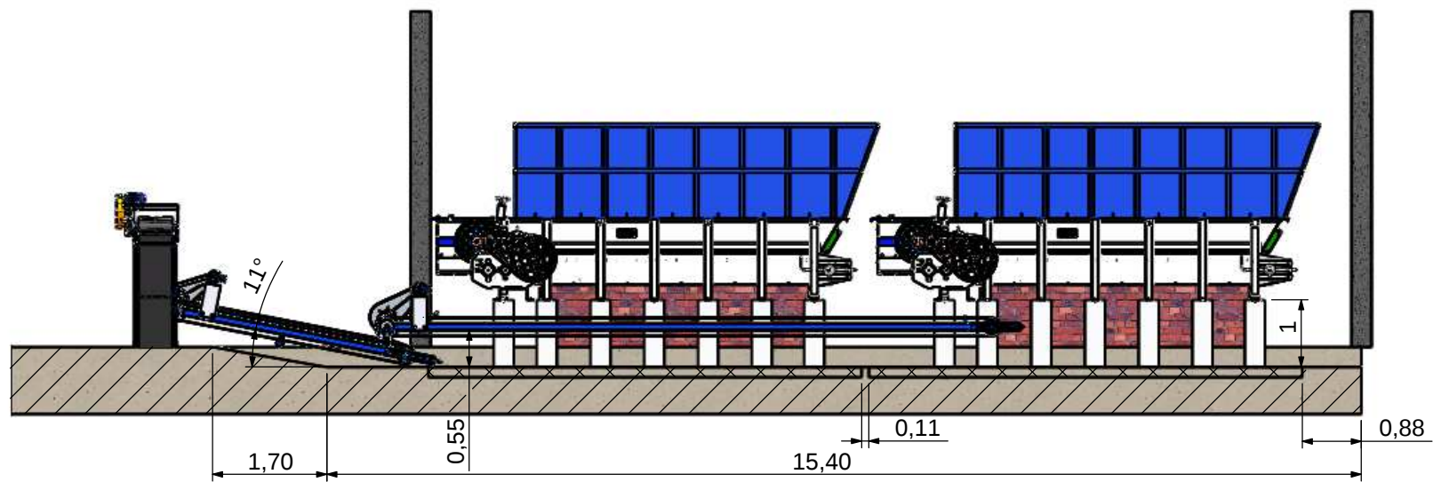
Vista em corte, para posicionamento dos caixões MN-6/1000.
