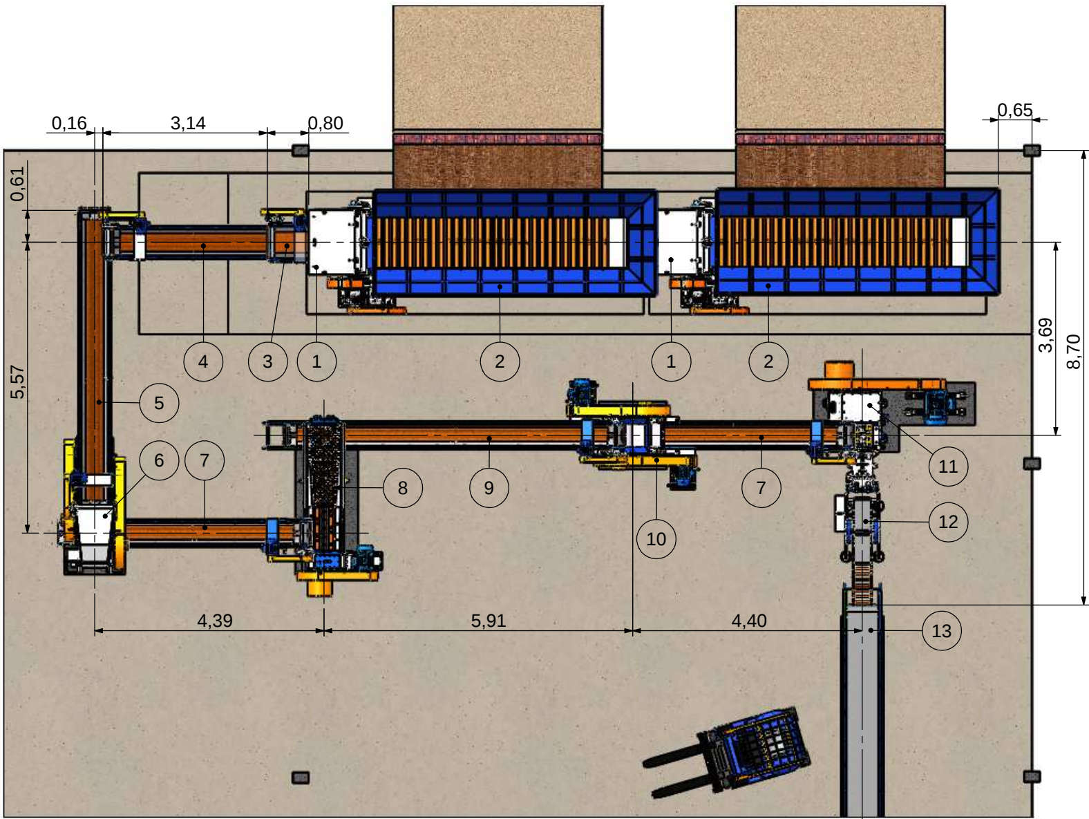
DETALHE A ESCALA 1 : 100
