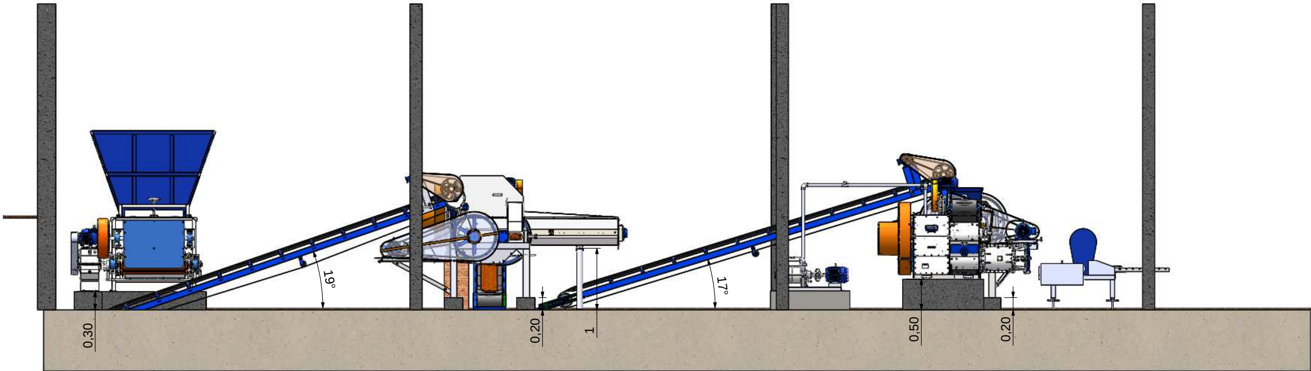
VISTA LATERAL
