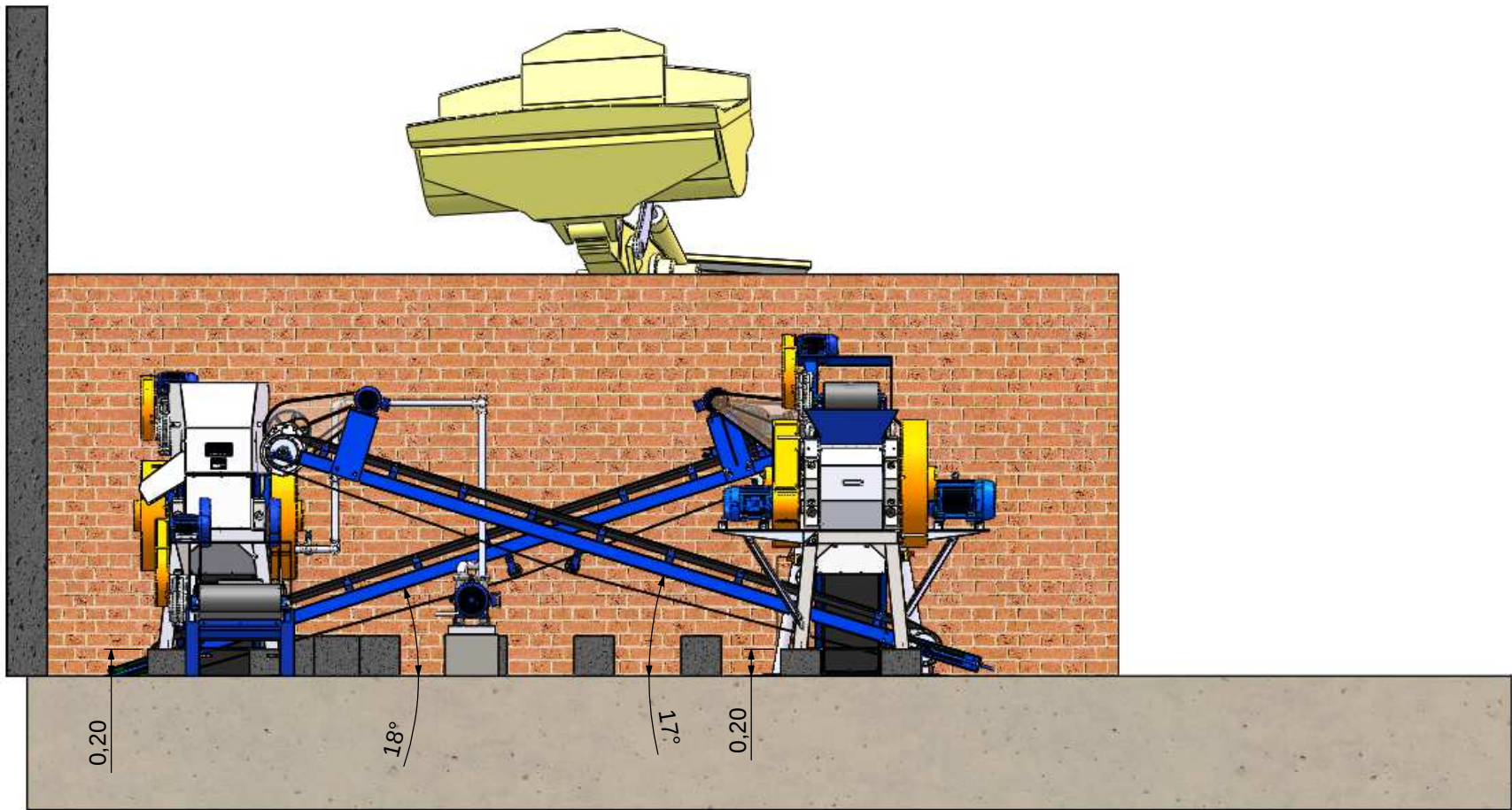
VISTA FRONTAL (Alguns componentes foram omitidos para melhor visualização)
